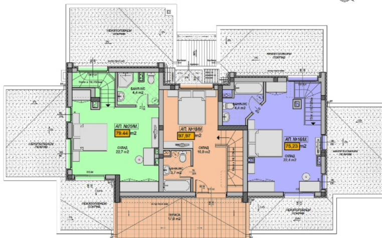
РАЗПРЕДЕЛЕНИЕ ТЕРАСОВИДЕН ЕТАЖ НА КОТА +11,20
