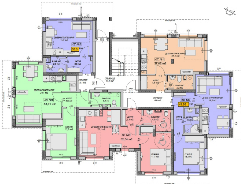
РАЗПРЕДЕЛЕНИЕ ПАРТЕР НА КОТА ±0,00
