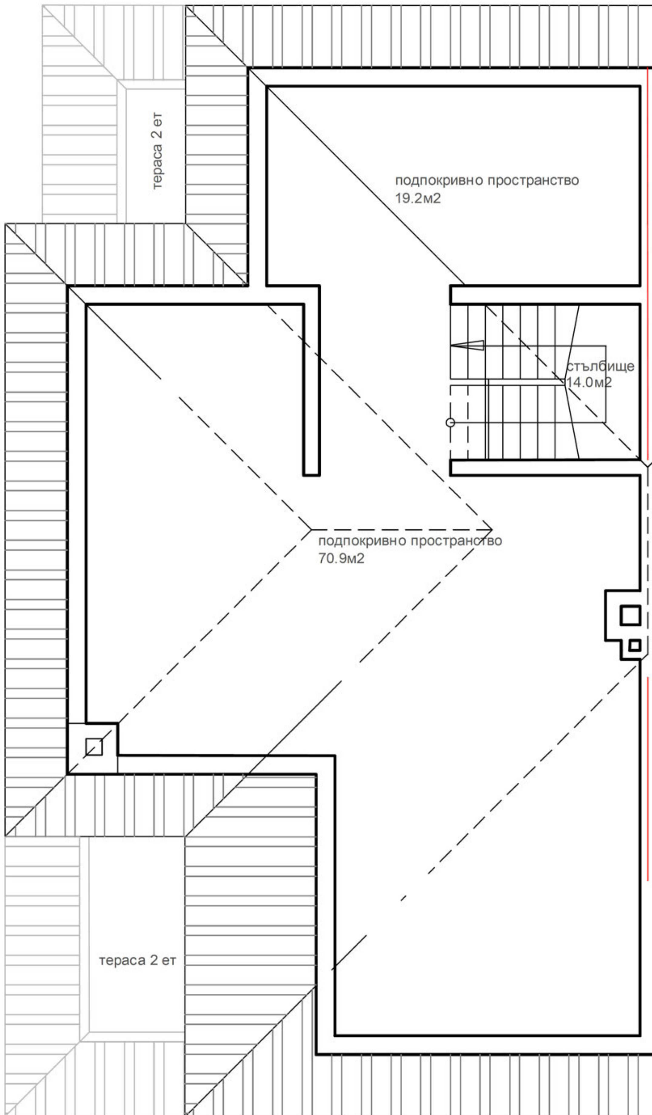
къща 4 разпределение трети етаж подпокривно пространство 120.1м2
