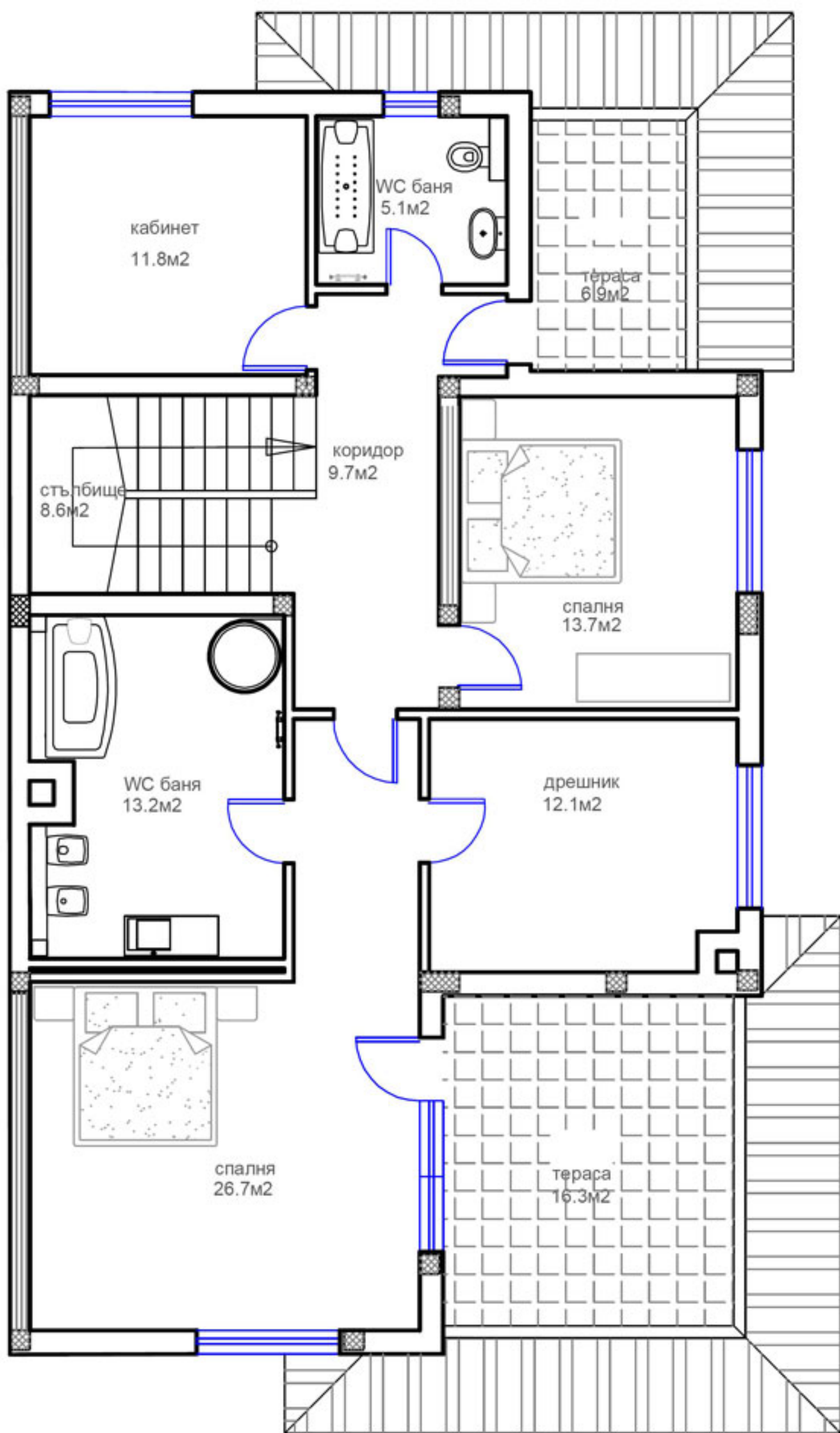
къща 9 разпределение втори етаж второ ниво=142.9 м 2
