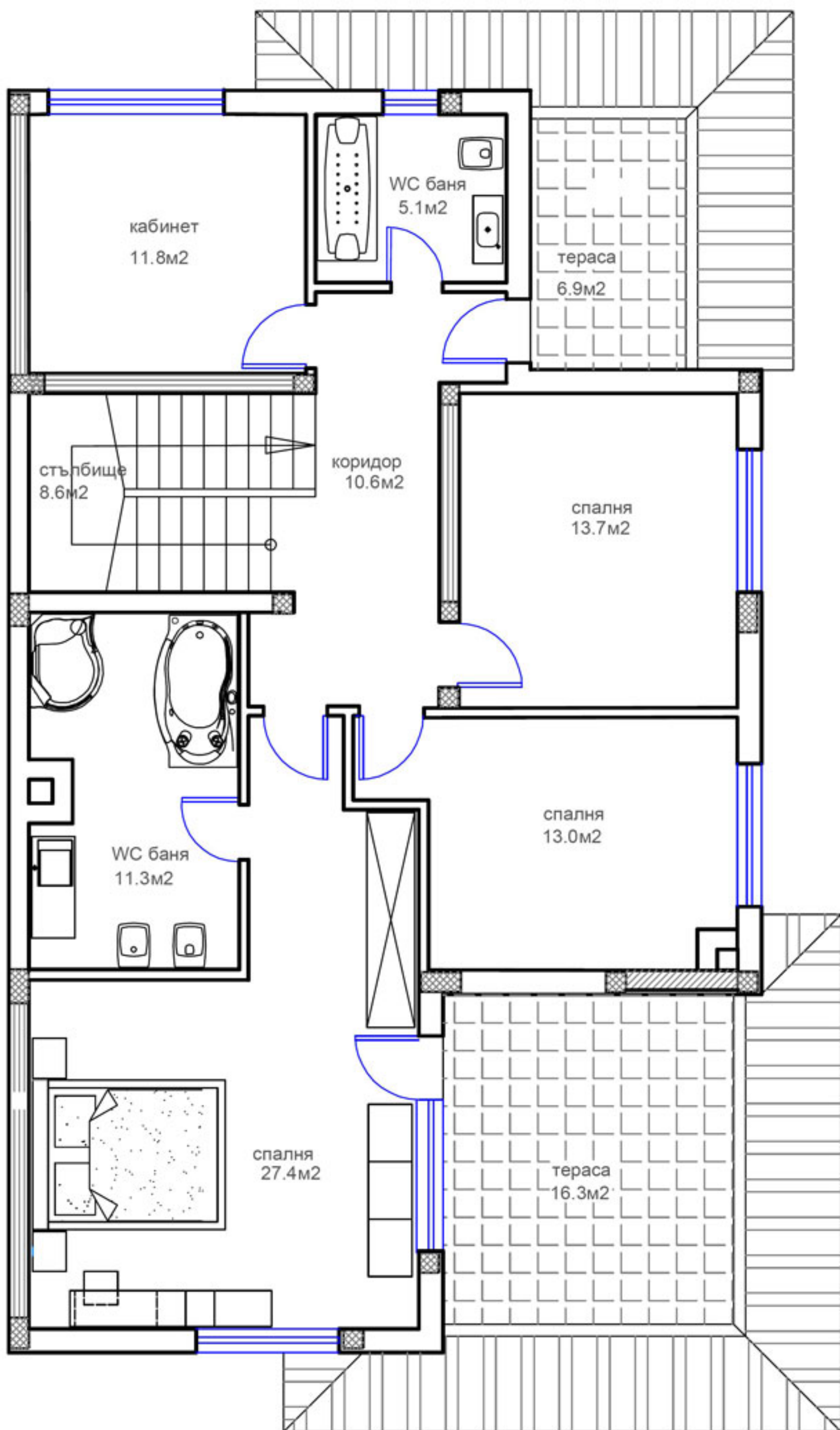
къща 3 разпределение втори етаж второ ниво=143м 2
