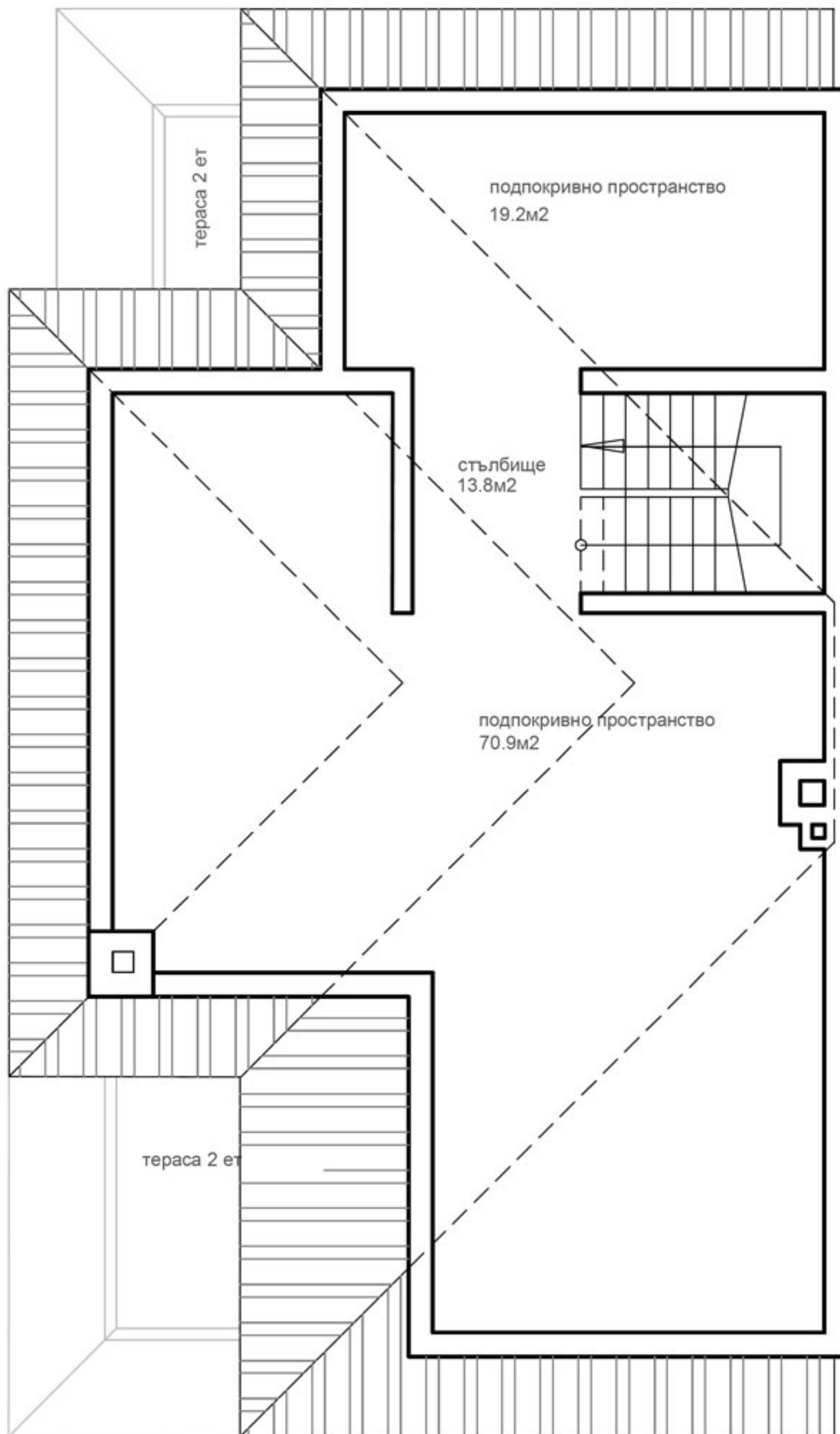
къща 8 подпокривно пространство 120.2м2
