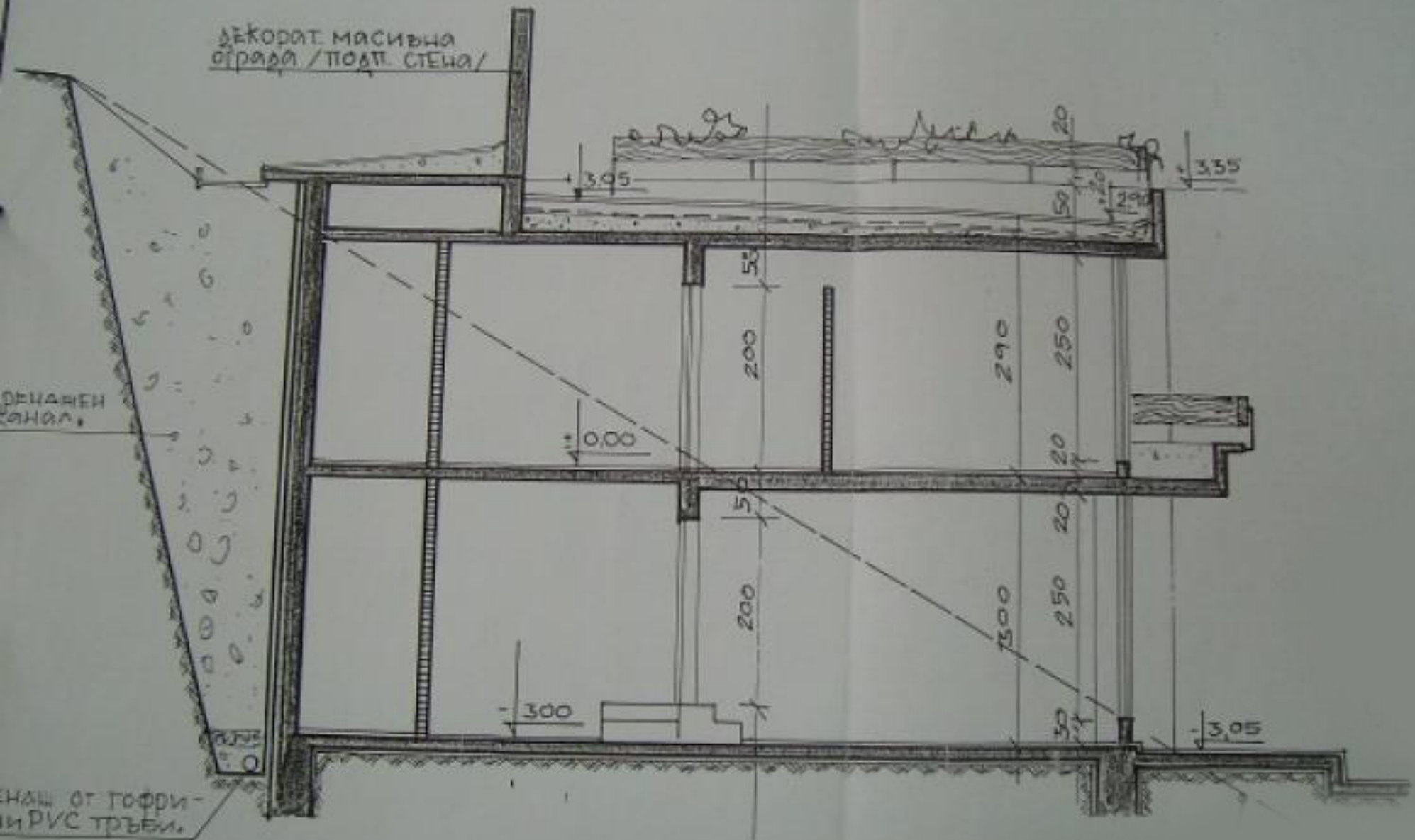
ВЕРТИКАЛЕН РАЗРЕЗ.
